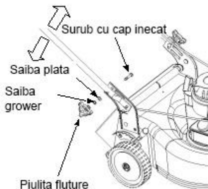
SL. 10 Piulita fluture-navrtka
